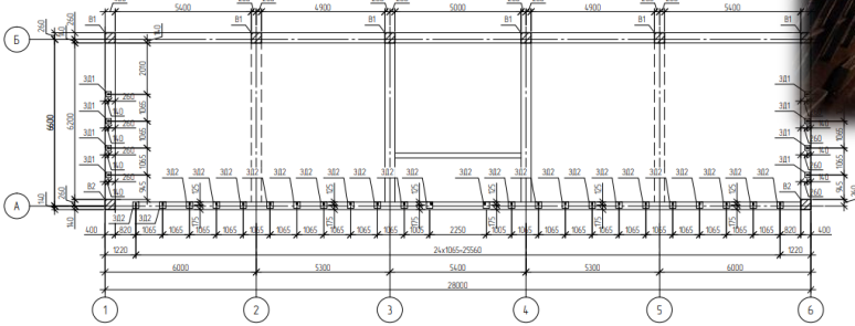
Схема размещения выпусков та закладних деталей фундаменту
